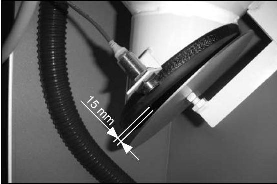
Abb. 29 Klappe offen Abstand Klappe-Dichtung , überprüfen und gegebenenfalls durch Verschieben des Gegengewichts Abstand auf 15 mm einstellen
