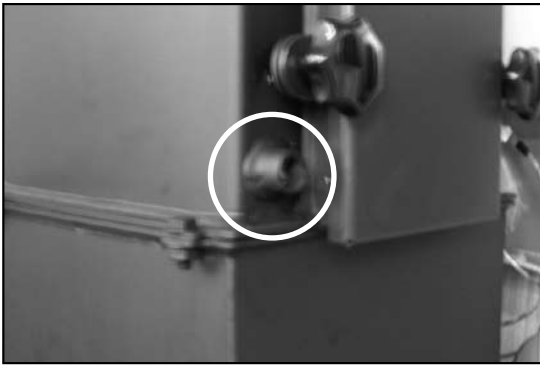
Abb. 08: Befüll- / Entleeranschluss BPH10, Anschluss 1/2 Zoll für KFE Hahn
