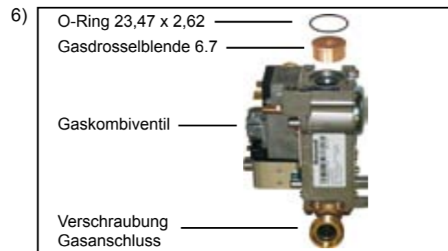
6) Verschraubung Gasanschluss mit O-Ring 26 x 4 an das neue Gaskombiventil für Flüssiggas anschrauben. Neue Gasdrosselblende mit Kennung 6.7 in Gaskombiventil einsetzen. Gaskombiventil mit O-Ring 23,4 x 2,6 an Mischkammer anschrauben.
