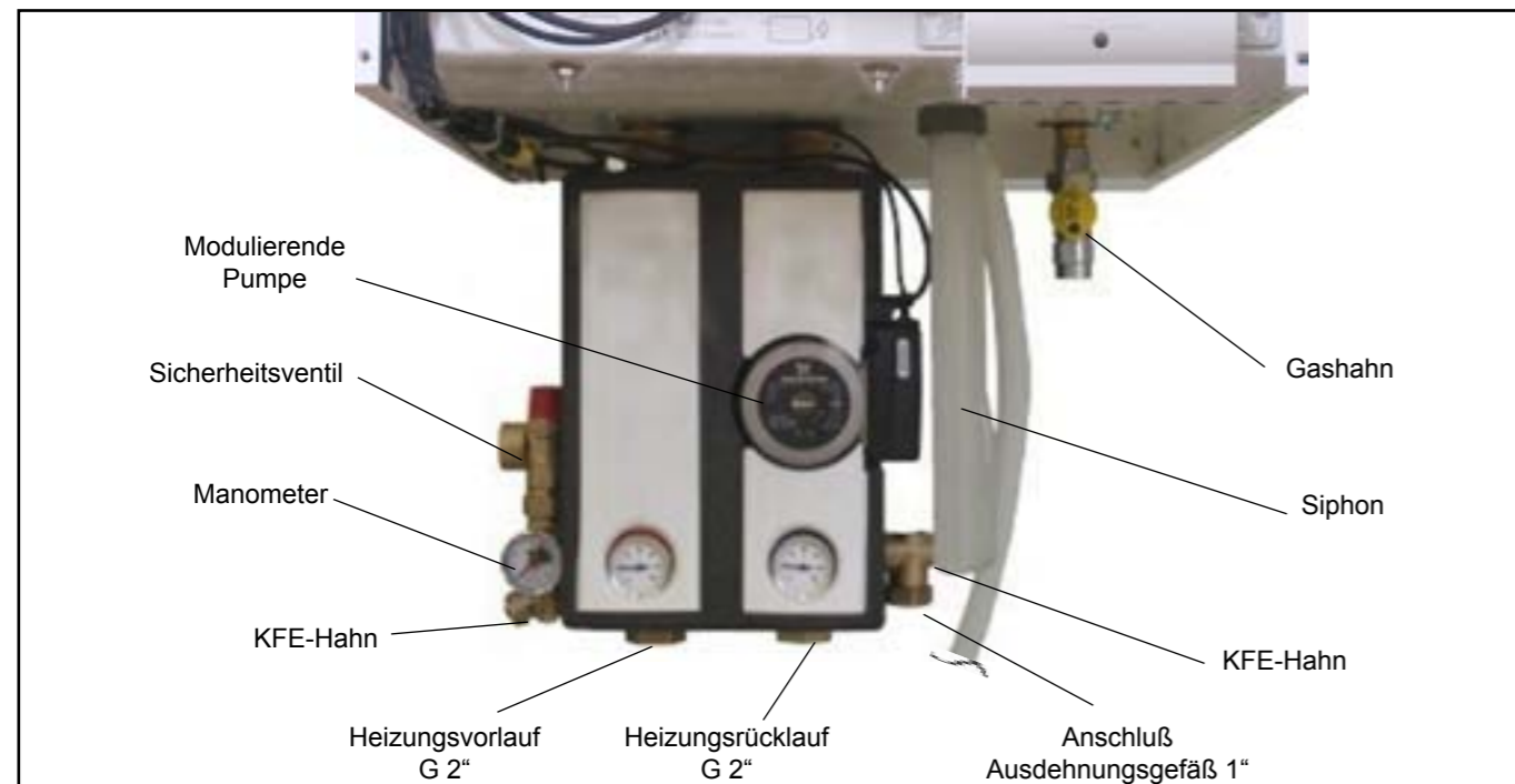
Bild: Pumpengruppe (Zubehör)
