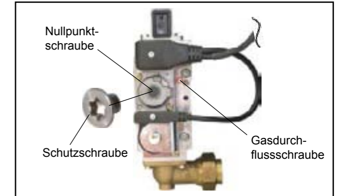
Bild: Gaskombiventil
