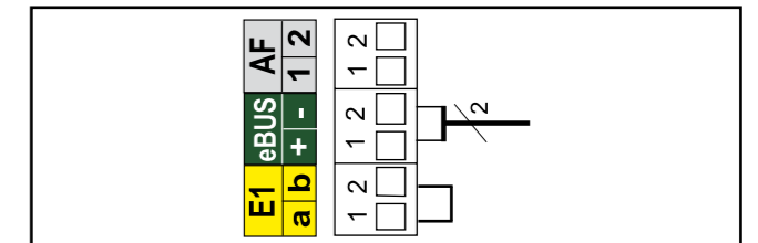
Bild: Anschluss Wolf-Regelungszubehör digital (eBus-Schnittstelle)
