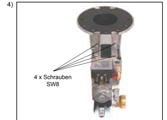
Gaskombiventil von der Mischkammer für Gas/Luft abschrauben (4 Schrauben SW8).
