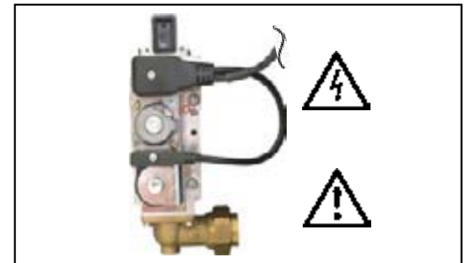
Bild: Gaskombiventil Gefahr durch elektrische Spannung Gefahr von Vergiftung und Explosion durch ausströmendes Gas
