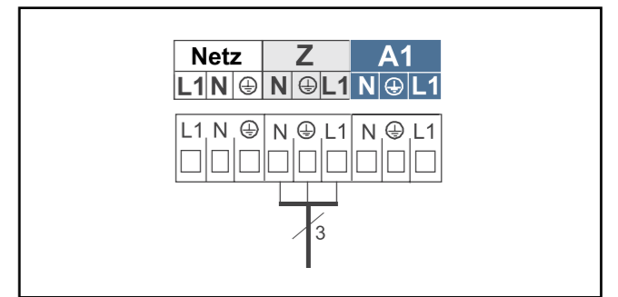
Bild: Anschluss Heizkreispumpe
