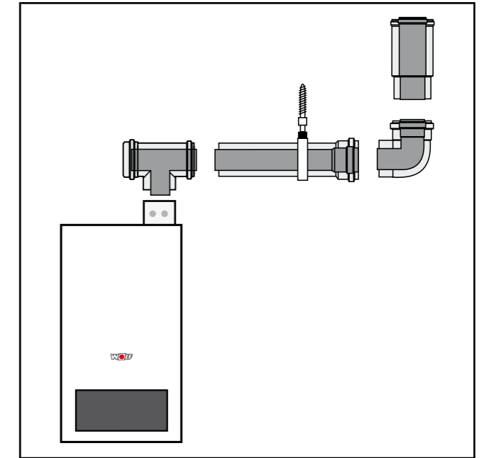
Bild: Beispiel Luft-/Abgasführung
