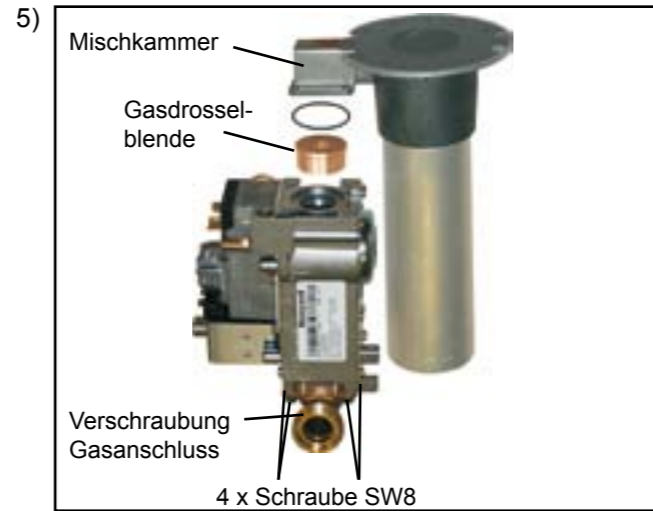
5) 4 Schrauben SW8 an der Verschraubung Gasanschluss entfernen und Verschraubung vom Gaskombiventil abnehmen. Gaskombiventil und Gasdrosselblende entfernen. Die Schutzkleber an Ventileinlass und Ventilauslass des neuen Gaskombiventils an die Öffnungen des entfernten Ventils anbringen.
