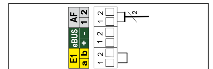
Bild: Anschluss Außenfühler
