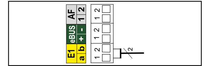
Bild: Anschluss Raumthermostat
