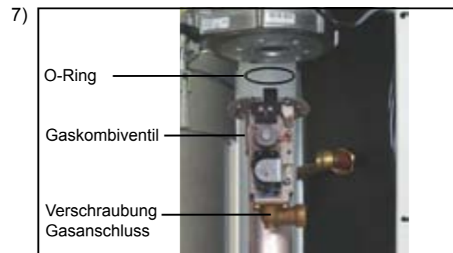
7) O-Ring mit Siliconfett in die Dichtnut des Gebläses heften und Mischkammer mit Gaskombiventil an Brennergebläse montieren. Verschraubung Gasanschluss mit Gaszuleitung dicht verschrauben.
