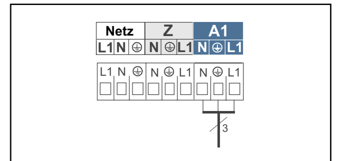
Bild: Anschluss Ausgang A1
