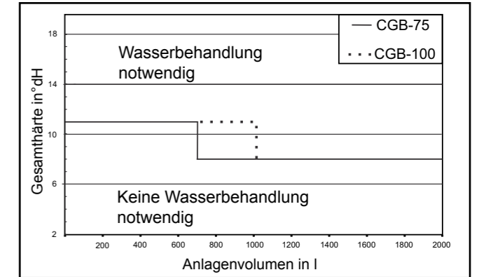
Diagramm: Wasserbehandlung
