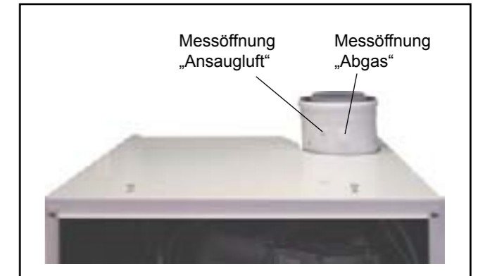
Bild: Messöffnungen
