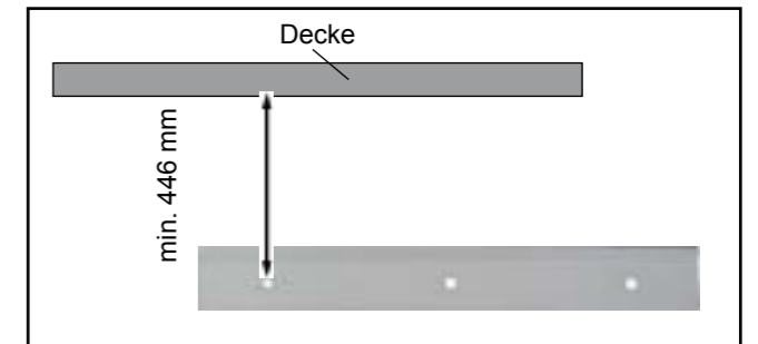
Bild: Bohrlöcher für Einhängewinkel
