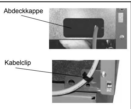
Bild: Brennerkabelbefestigung
