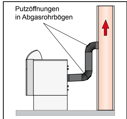
Bild: Putzöffnungen
