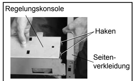
Bild: Montage Regelungskonsole
