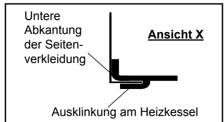
Bild: Montage Seitenverkleidung
