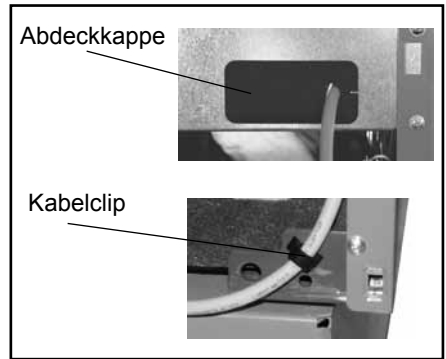
Bild: Brennerkabelbefestigung
