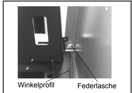
Bild: Montage Seitenverkleidung
