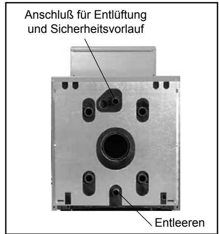
Bild: Entleeren der Heizungsanlage
