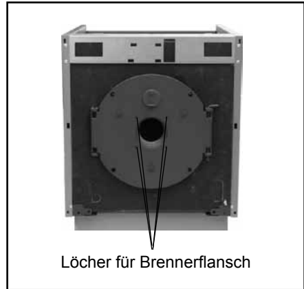
Bild: Kesselflansch
