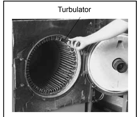
Bild: Turbulatoren
