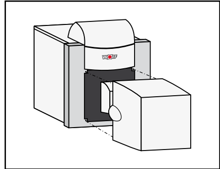
Bild: Montage „Große Schalldämmhaube“
