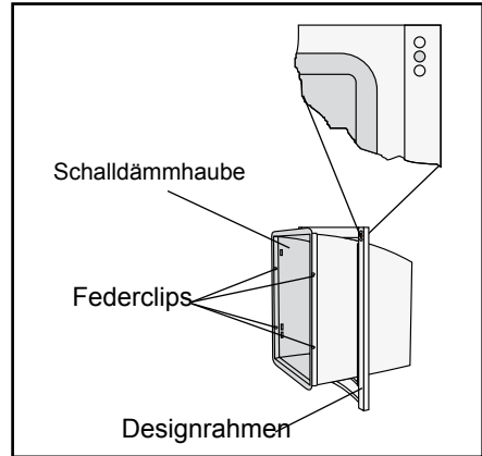
Bild: Schalldämmhaube in Designrahmen einclippen
